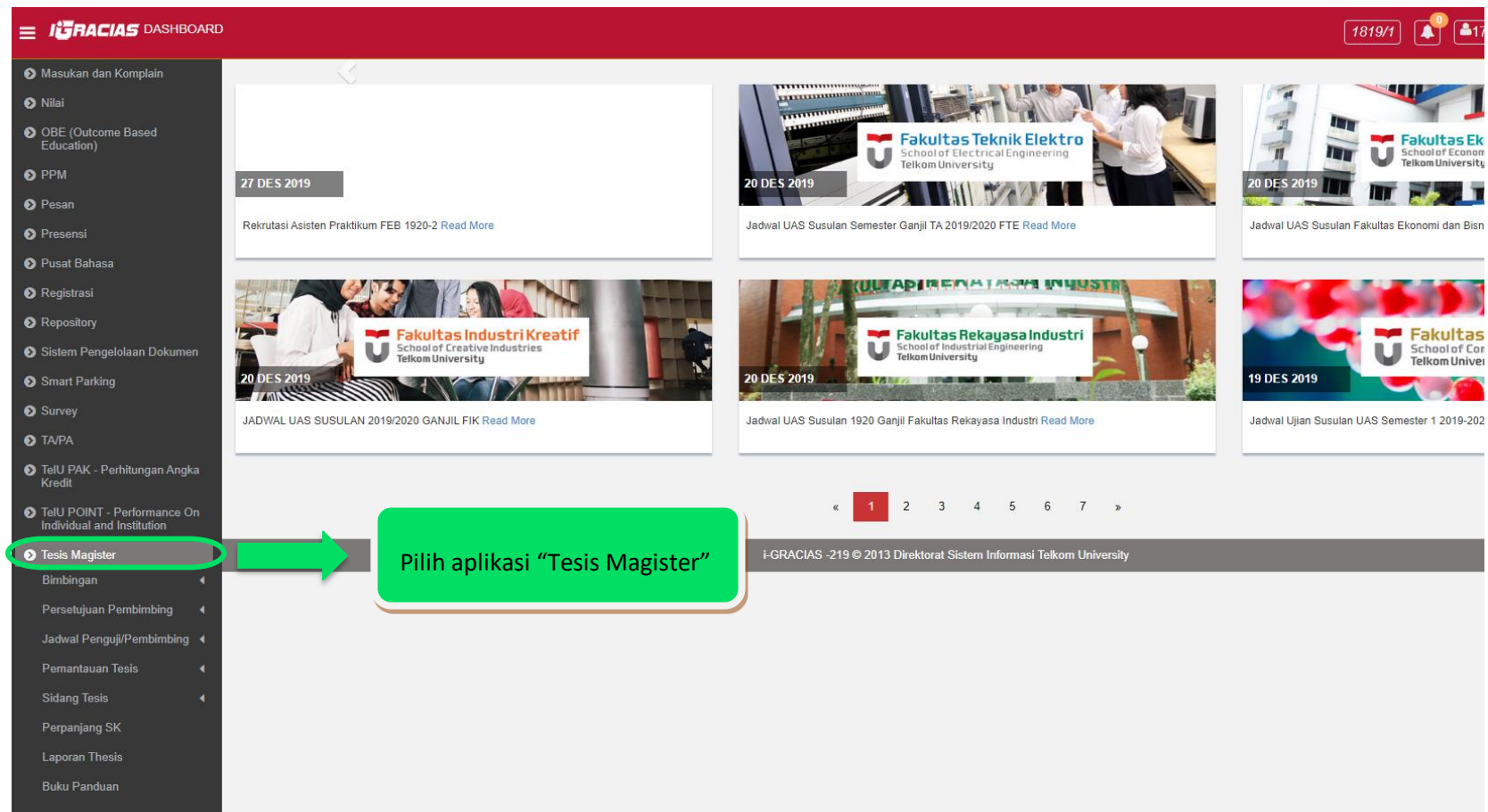
Gambar 1 Dashboard iGracias
